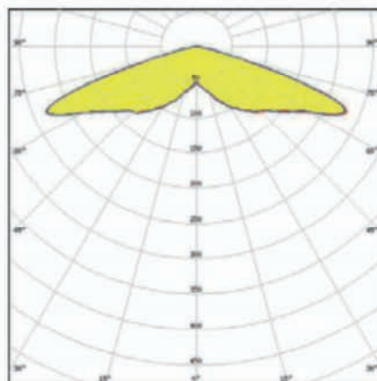
ASIMÉTRICA EXTENSIVA
