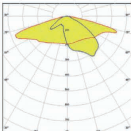
ESTANDAR 120º
