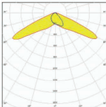
ASIMETRICA LONGITUDINAL
